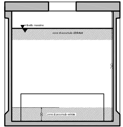
sezione trasversale
