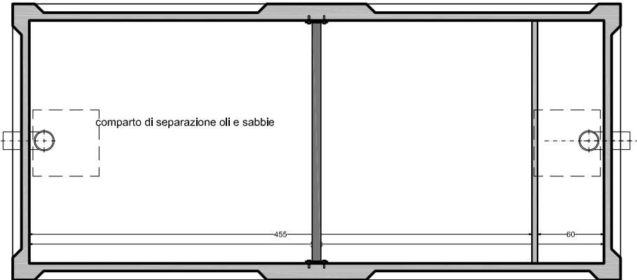
pianta copertura
